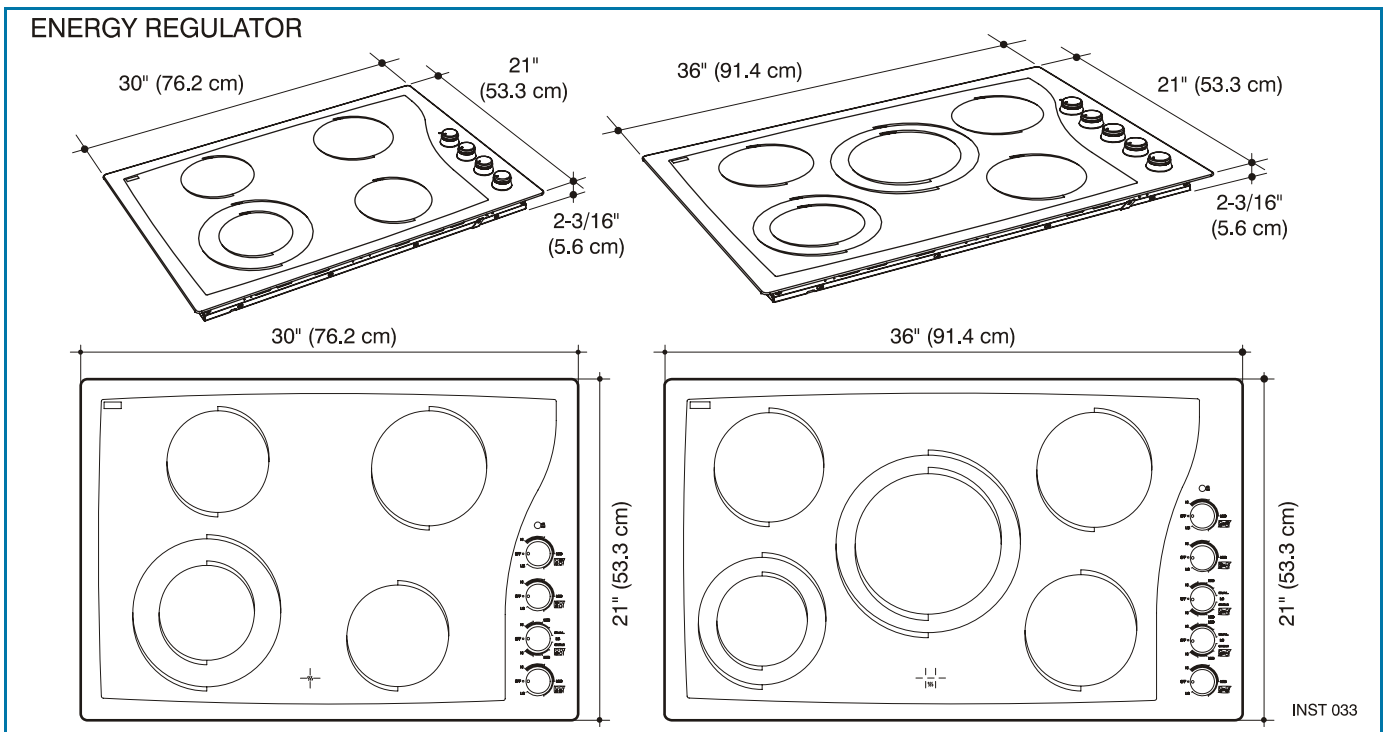
Figura 2. Regulador de energía (Energy Regulator)
